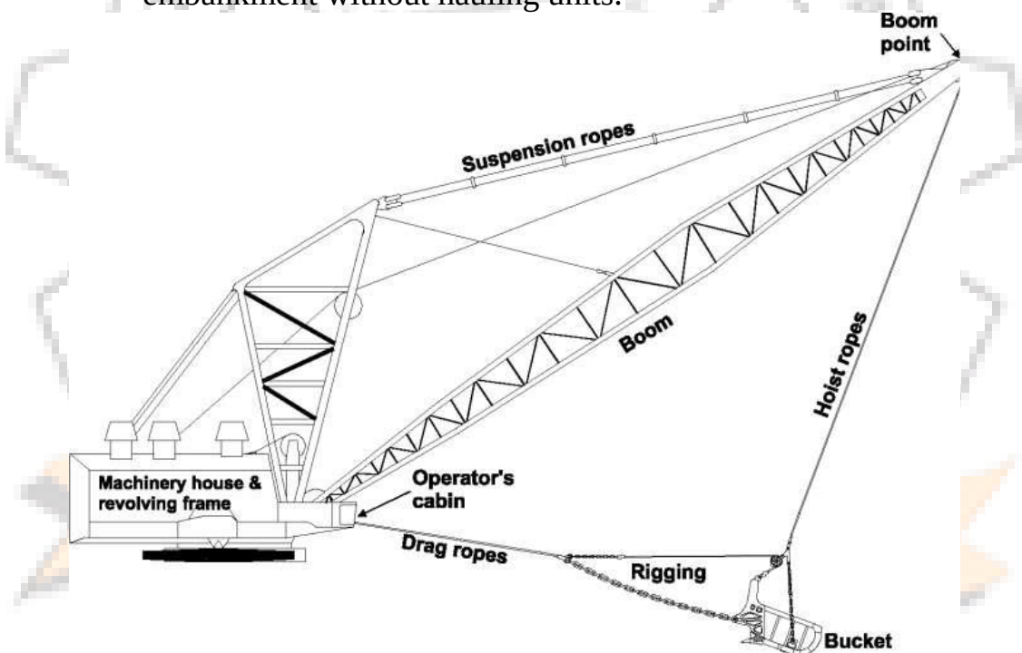
Fig. Dragline
