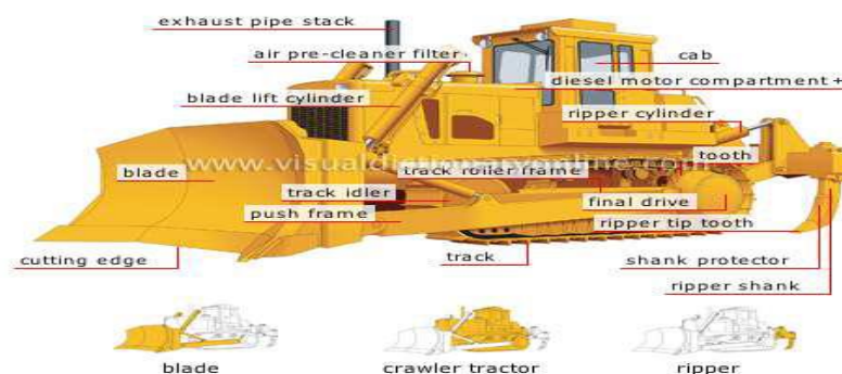
Fig. Bulldozer
