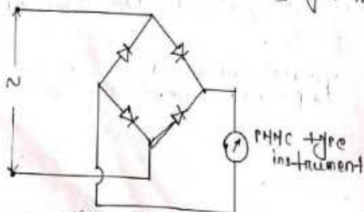
Fig: Rectifier (full wave bridge) type instrument
