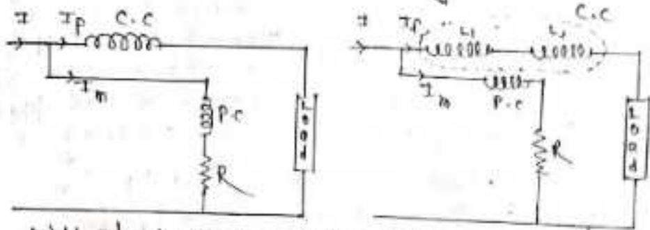
Fig: Electrodynamometer type wattmeter.
