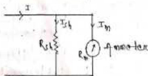
Fig: Basic ammeter
