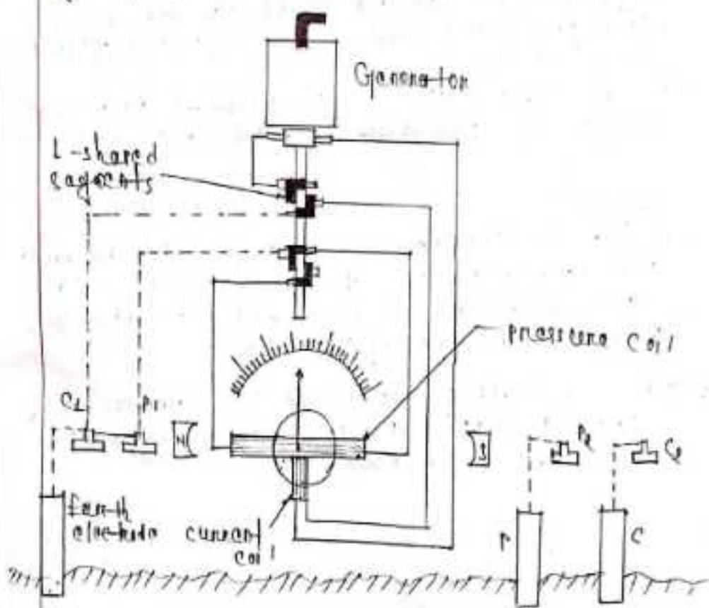
Fig: Earth tester.
