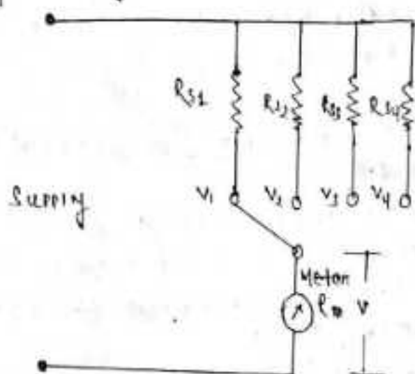
Fig: Multi-range voltmeter
